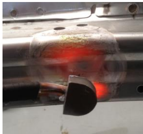
Richten des Längsträgers (außer hochfester Stahl)
